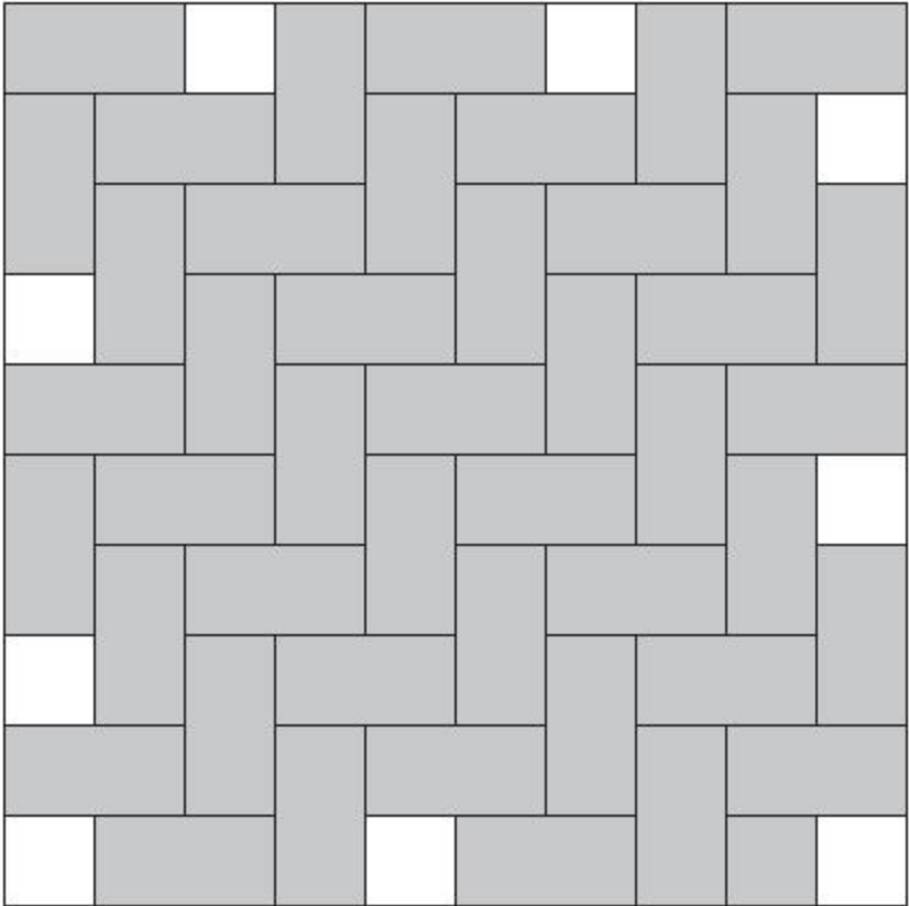
Rechteckpflaster Fischgrät
