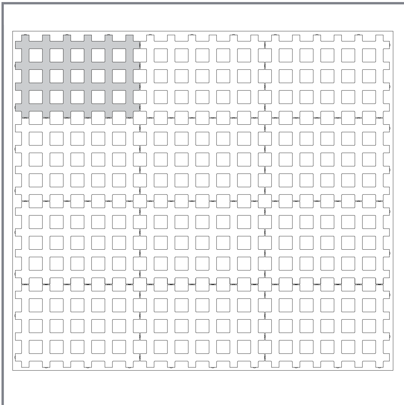
Verlegemuster HP001
