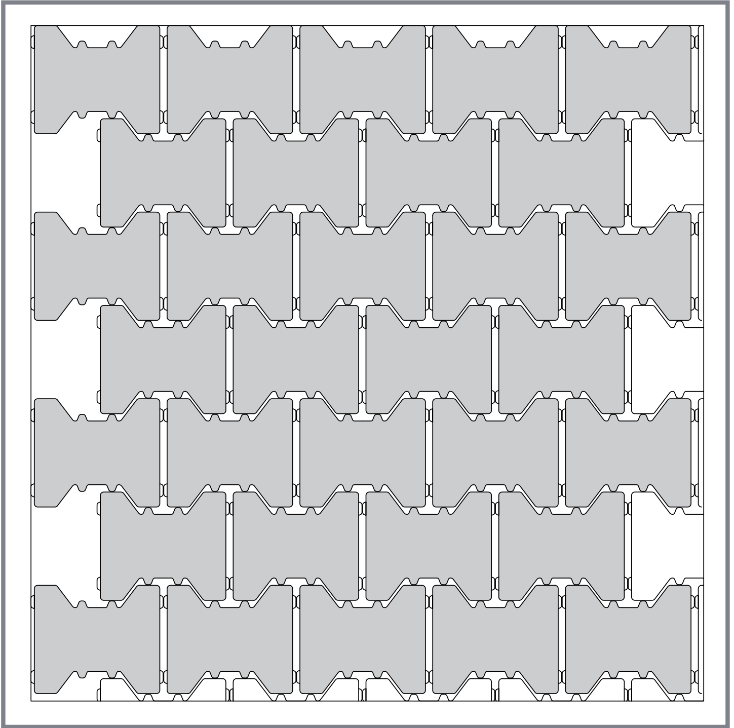
Verlegemuster DD001
