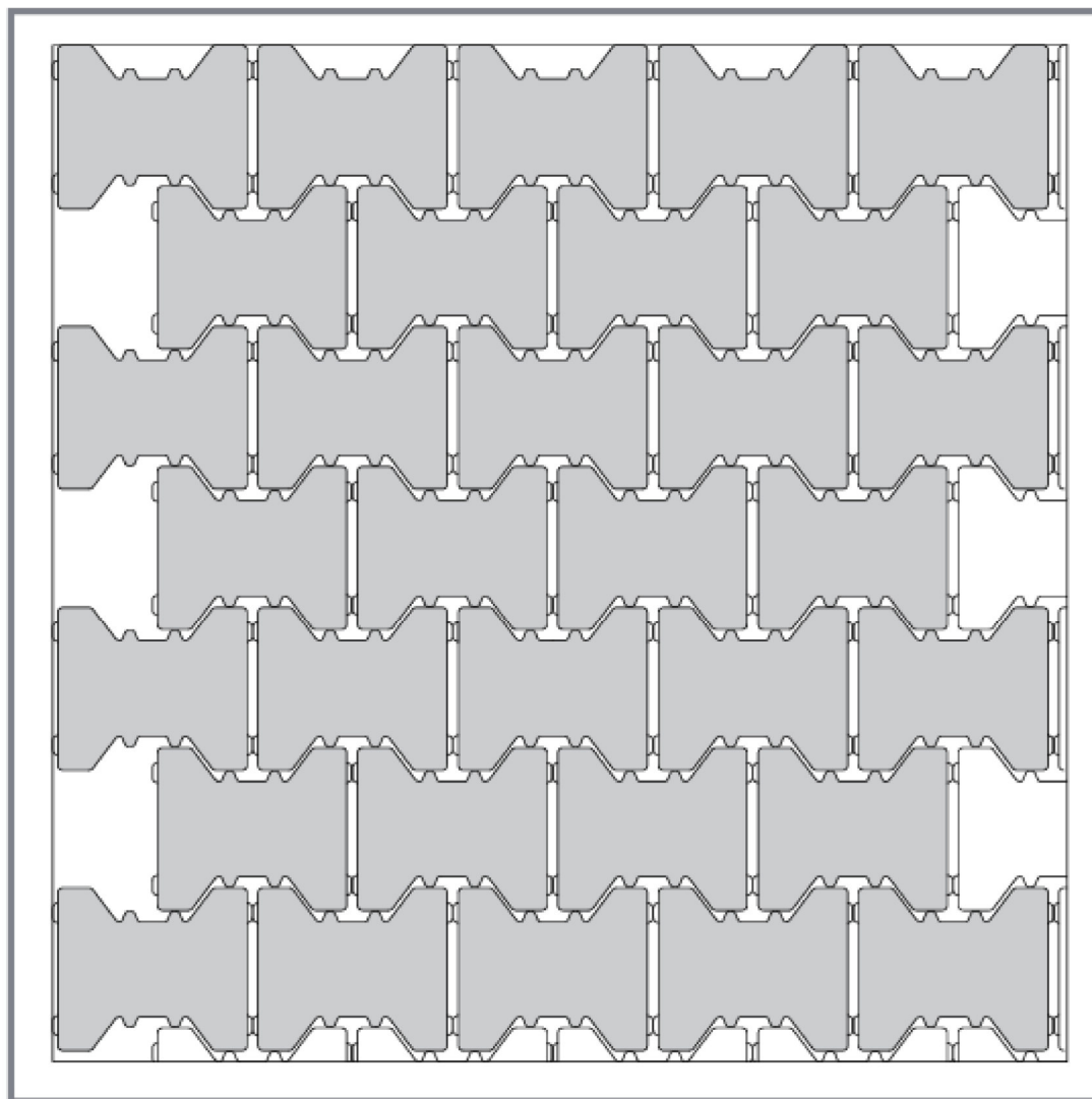
Verlegemuster DD001
