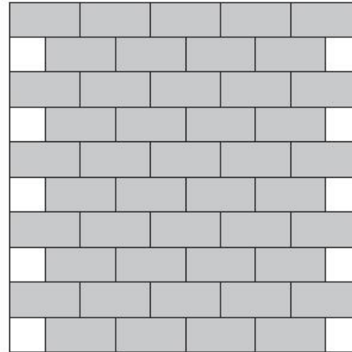
Rechteckpflaster Halbverband
