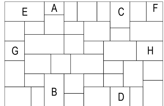
Verlegeeinheit = 0,96 m 2
