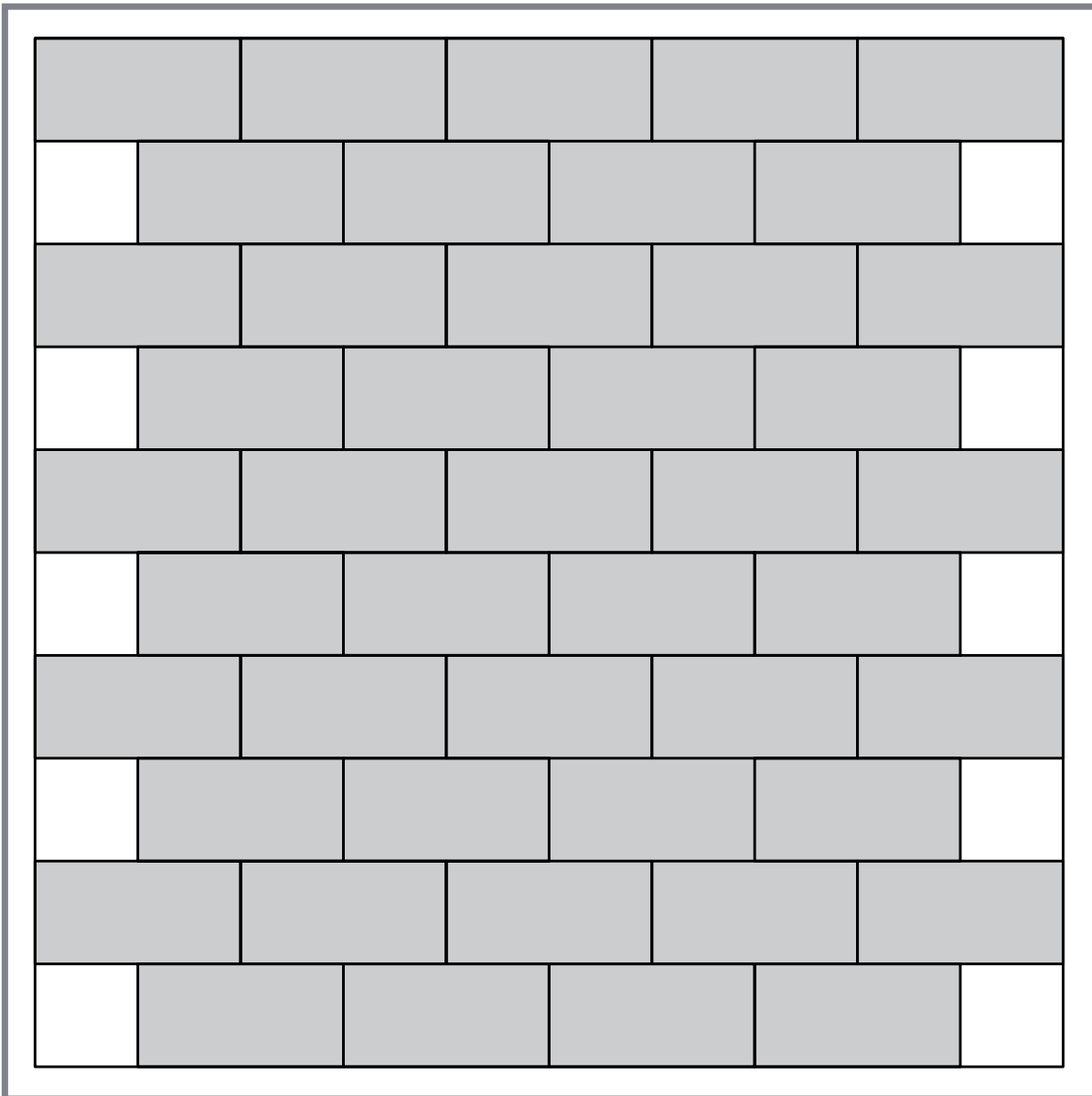
Verlegemuster RE001
