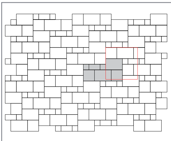
Verlegemuster HA002
