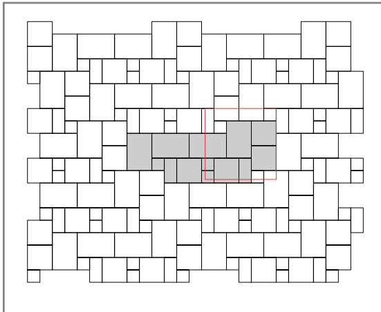
Verlegemuster HA001
