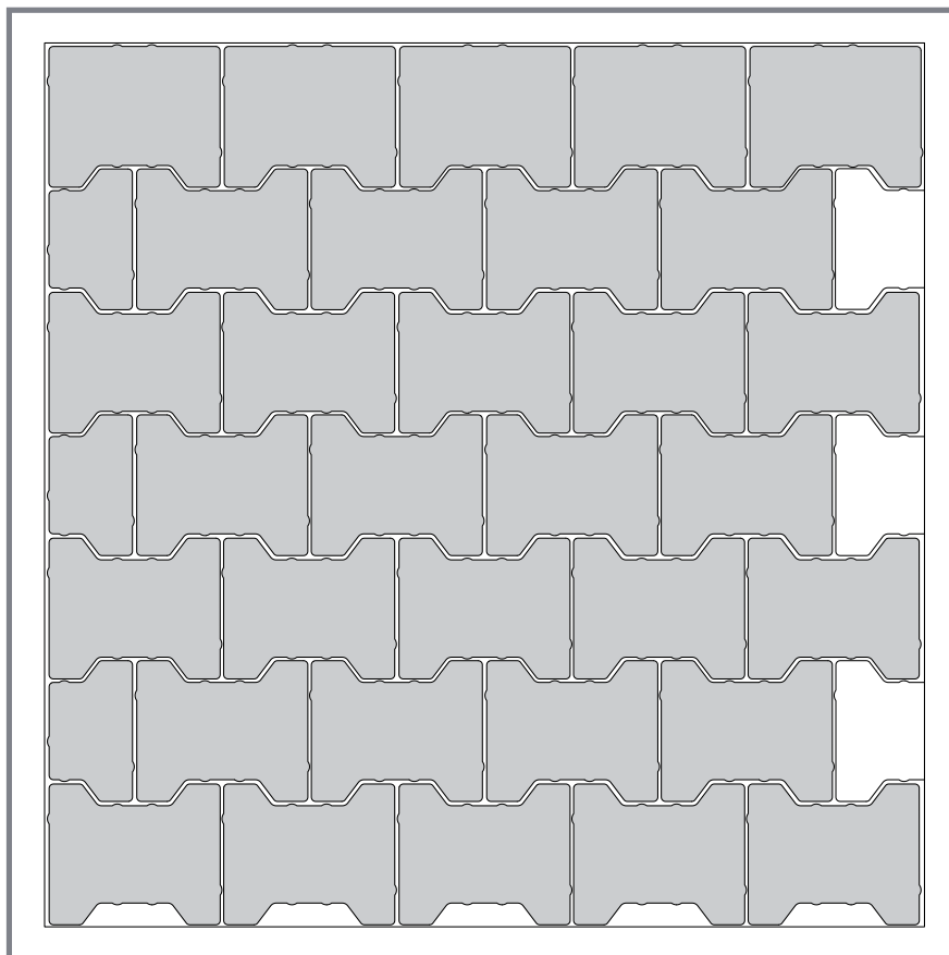
Verlegemuster DV001
